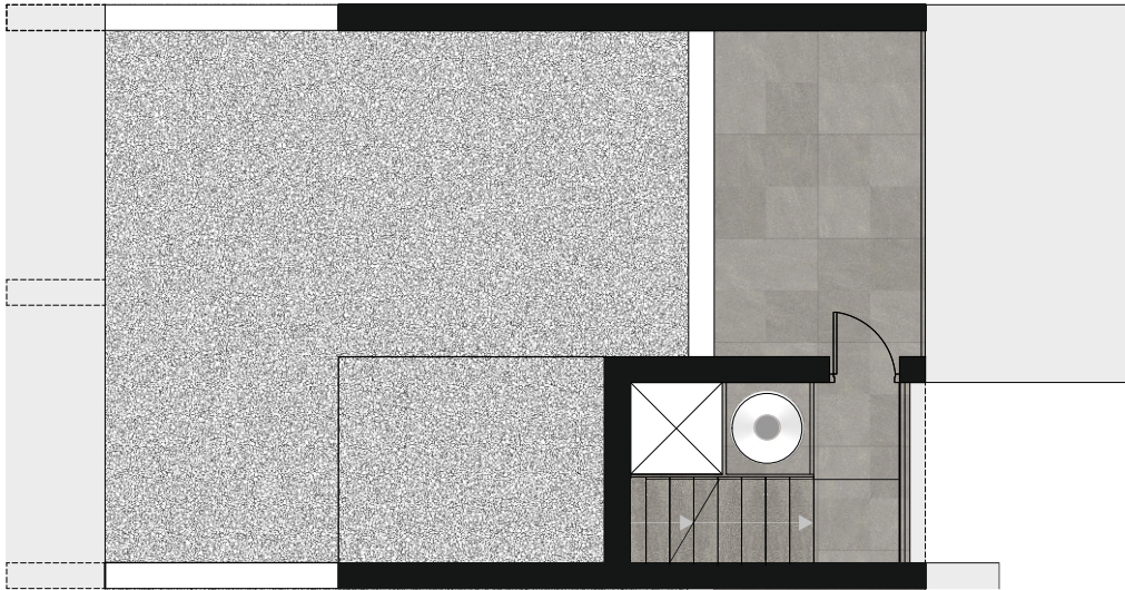
Planta alta
